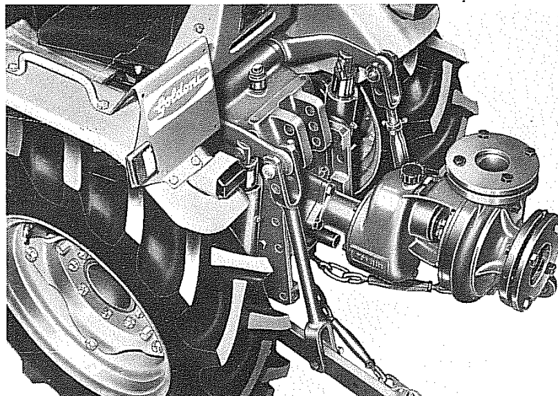
Fig. 104 - Pompa centrifuga
