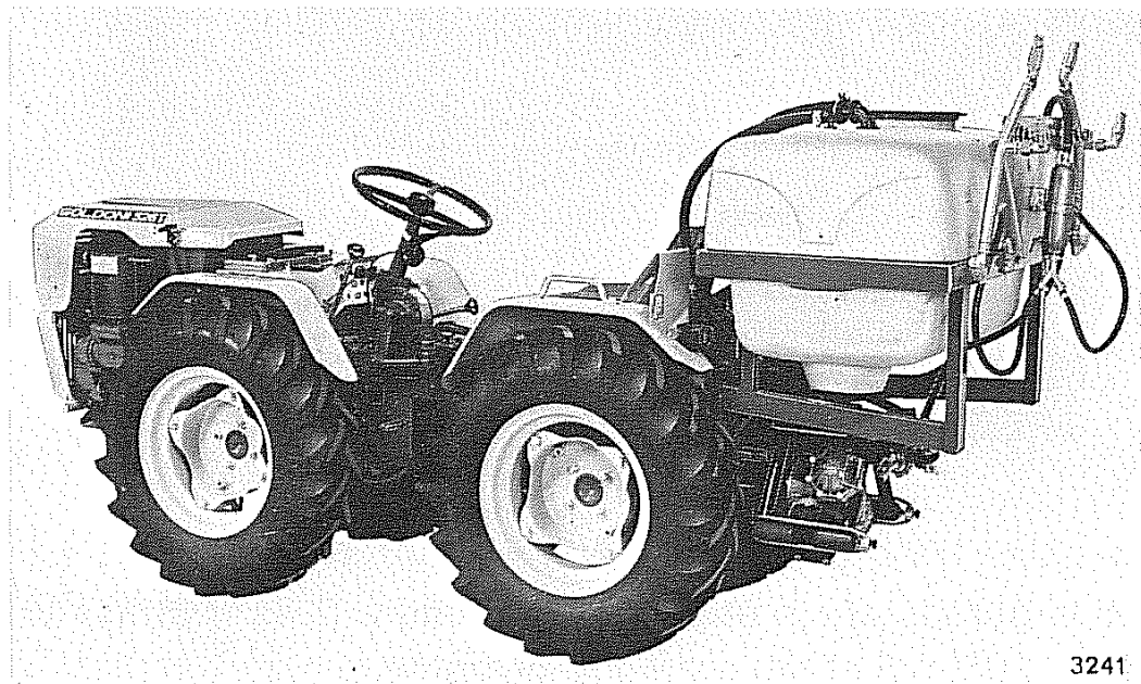
Fig. 100 - Gruppo irrorante
