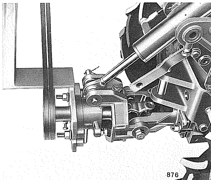
Fig. 71 - Attacco sega circolare
