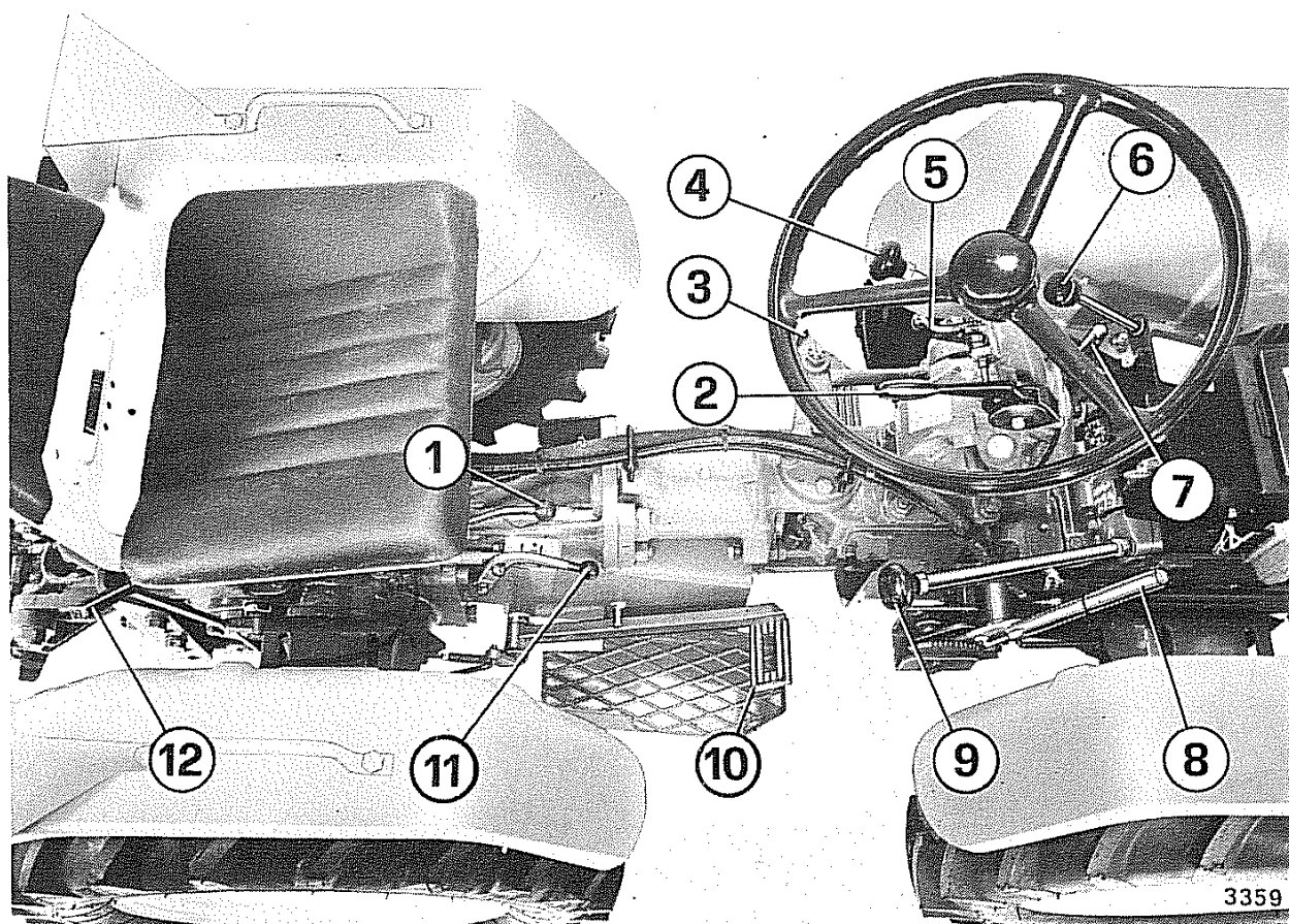
Fig. 1 - Comandi
