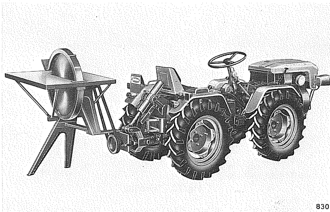
Fig. 70 - Sega circolare
