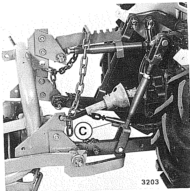
Fig. 107 - Attacco falciatrice laterale
