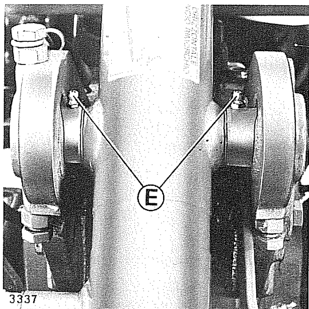
Fig. 22 - Punti d'ingrassaggio
