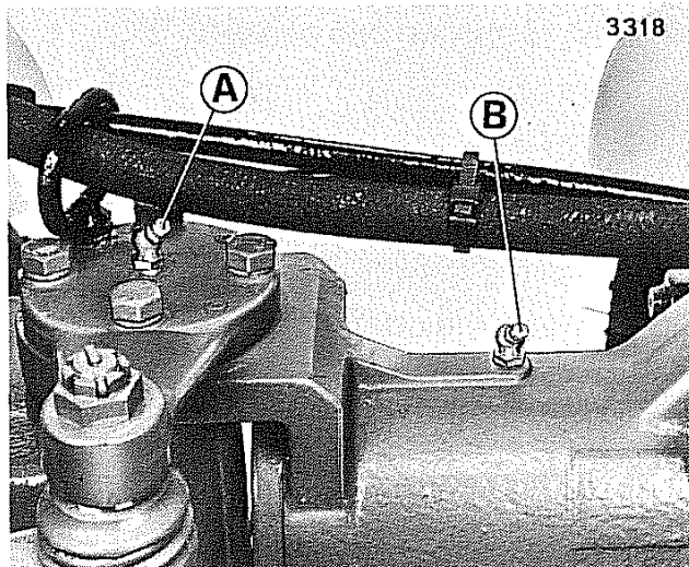
Fig. 19 - Punti d'ingrassaggio
