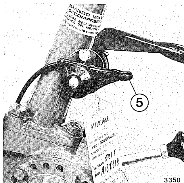
Fig. 17 - Comando valvola di decompressione.
