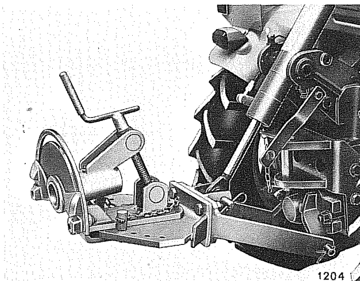
Fig. 59 - Porta aratri mod. "PH17"
