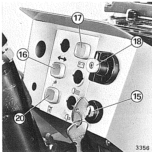
Fig. 5 - Strumentazione cruscotto (per mod. 526T e 530T).
