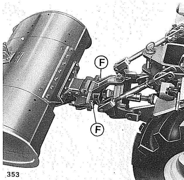
Fig. 75 - Fresa tipo "28"
