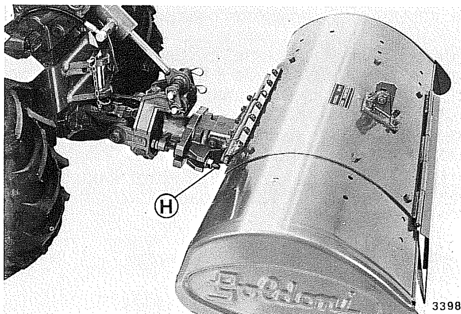
Fig. 45 - Fresa tipo "28"
