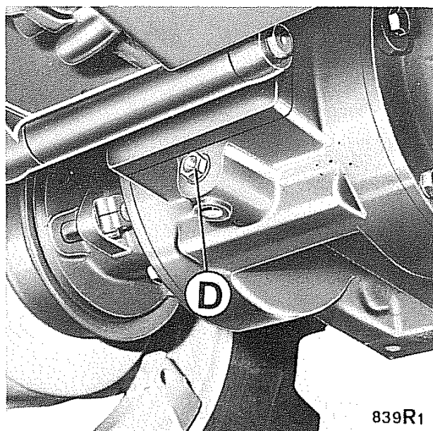
Fig. 26 - Scarico olio nel differenziale posteriore
