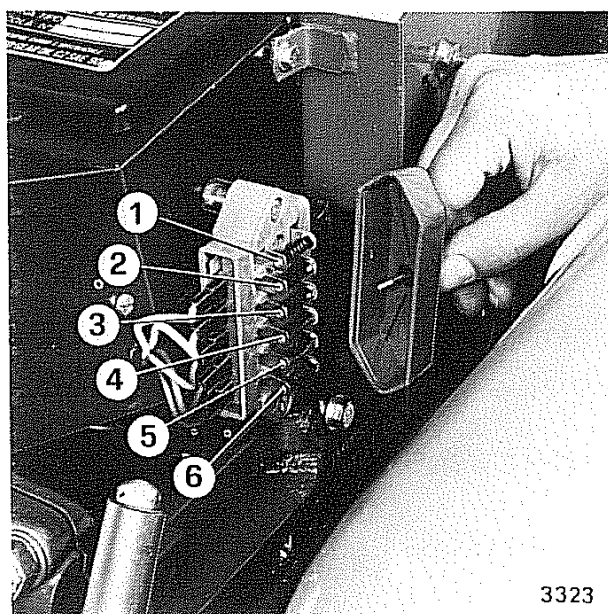
Fig. 34 - Valvole fusibili per mod. 520T e 521T
