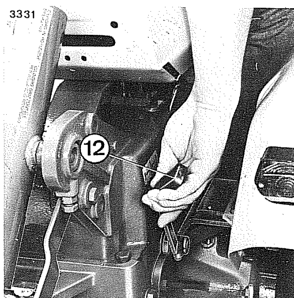
Fig. 9 - Bloccaggio differenziale posteriore
