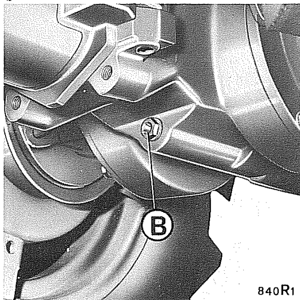
Fig. 24 - Scarico olio nel carter cambio
