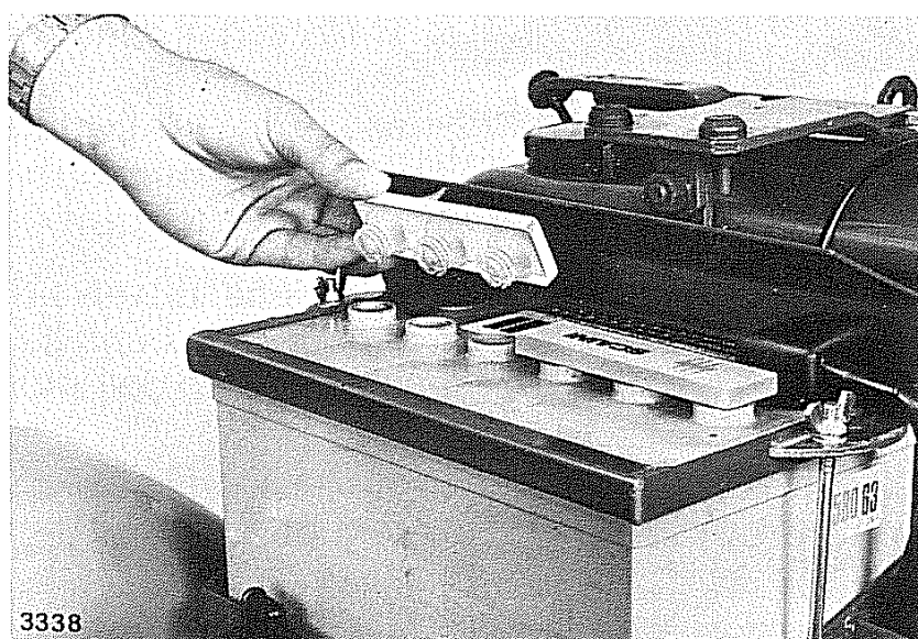
Fig. 33 - Controllo livello dell'elettrolita
