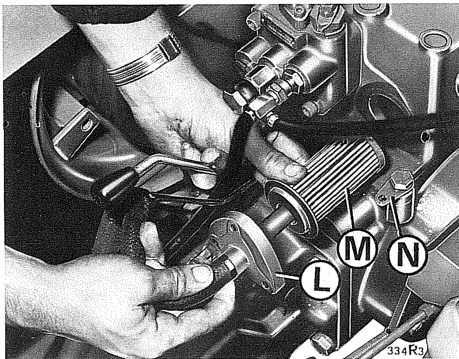
Fig. 32 - Pulizia filtro olio idraulico
