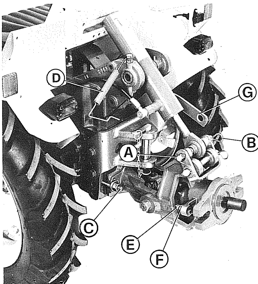
Fig. 44 - Snodo fresa
