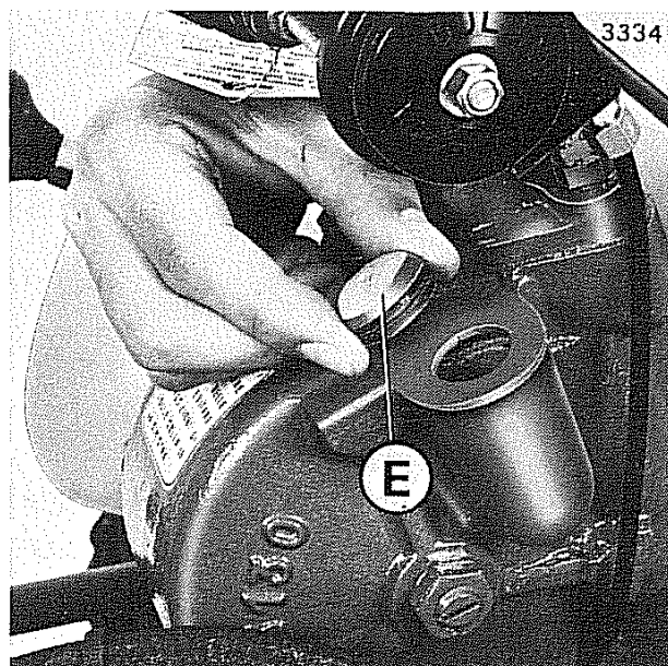
Fig. 27 - Sostituzione olio nella scatola sterzo
