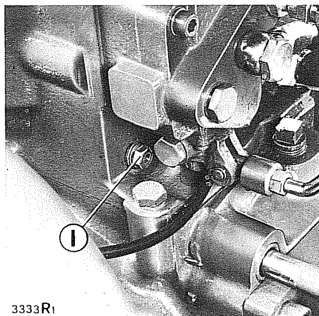
Fig. 31 - Scarico olio nei sollevatori
