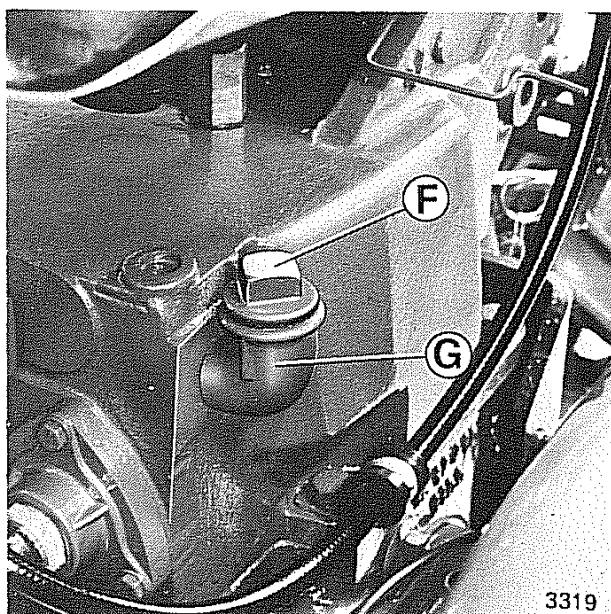
Fig. 28 - Immissione e livello olio nel sollevatore a 2 punti.
