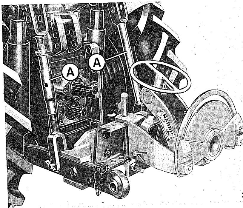
Fig. 83 - Porta aratri mod. "P13"
