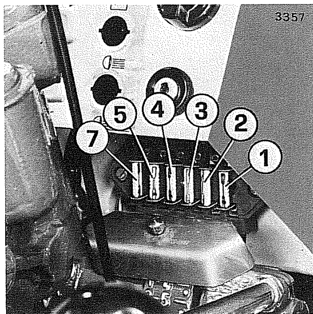
Fig. 35 - Valvole fusibili per mod. 526T e 530T
