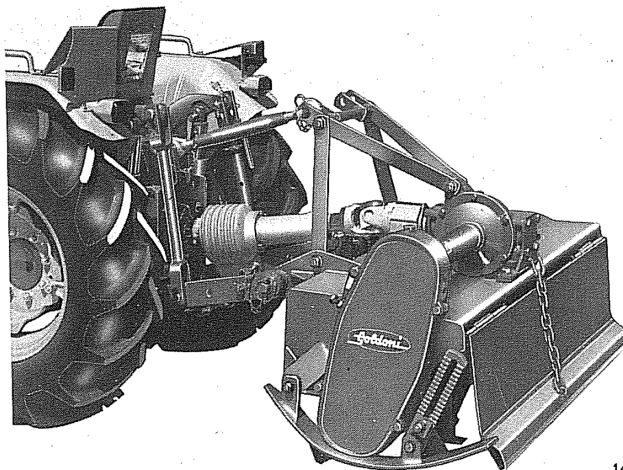
Fig. 76 - Fresa tipo "40"
