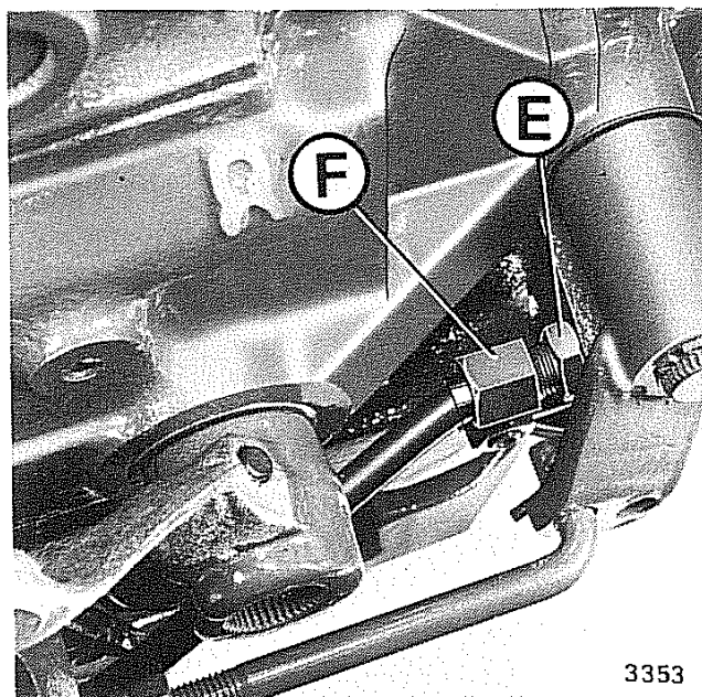
Fig. 38 - Registrazione frizione
