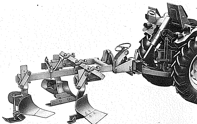
Fig. 58 - Aratro polivomere mod. "VR13"
