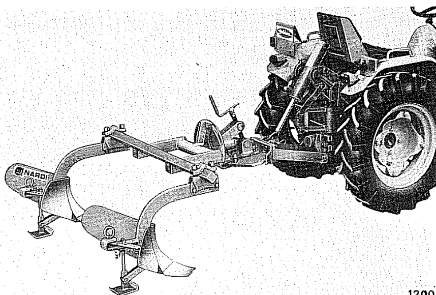
Fig. 57 - Assolcatore-Rincalzatore mod. "2AS13"
