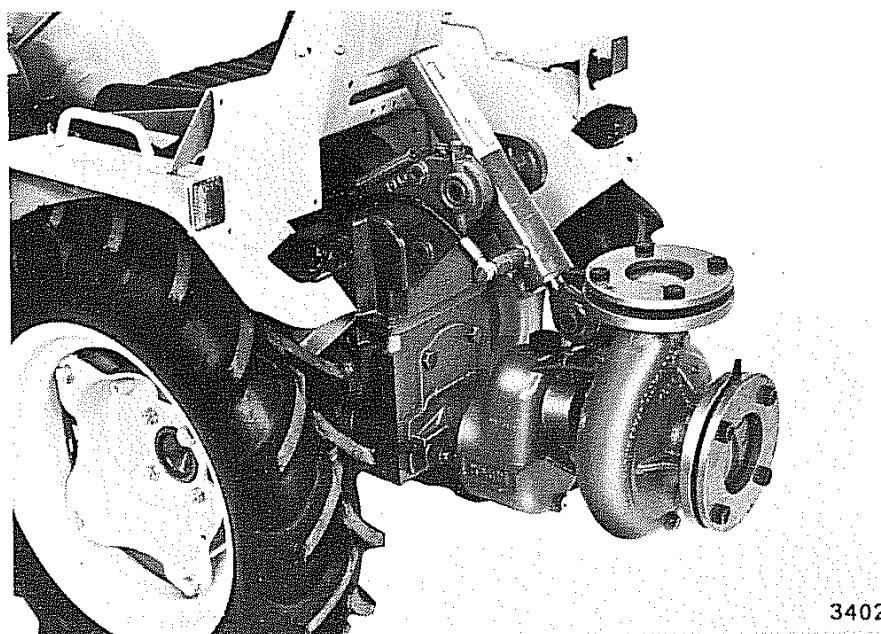
Fig. 63 - Pompa centrifuga
