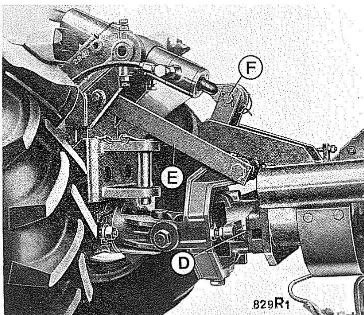
Fig. 69 - Attacco falciatrice laterale
