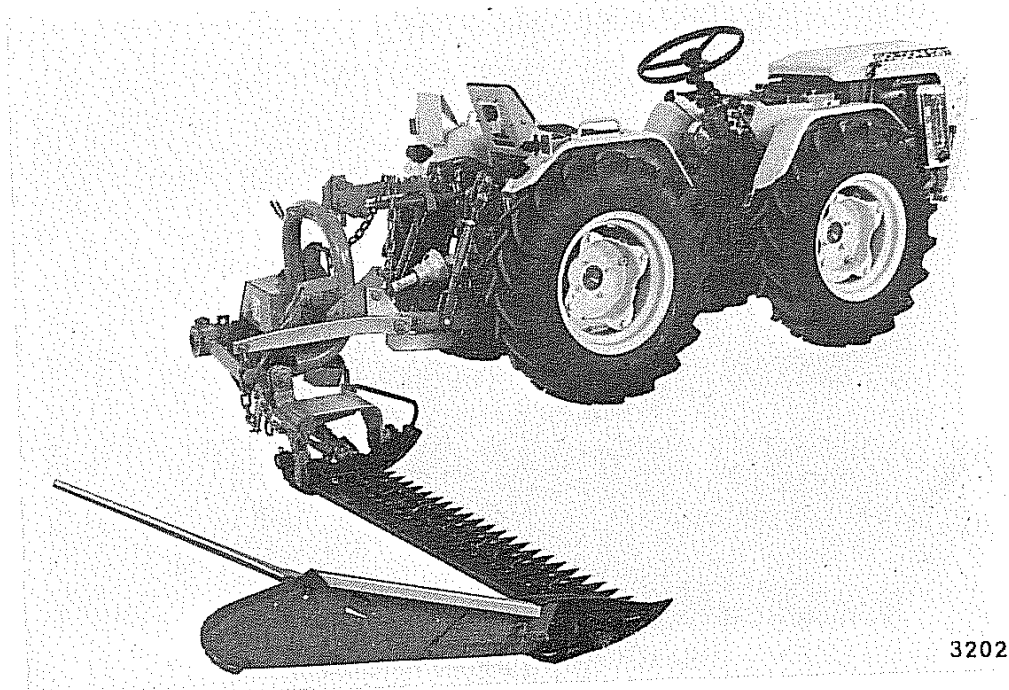
Fig. 106 - Falciatrice laterale
