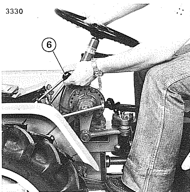
Fig. 8 - Bloccaggio differenziale anteriore
