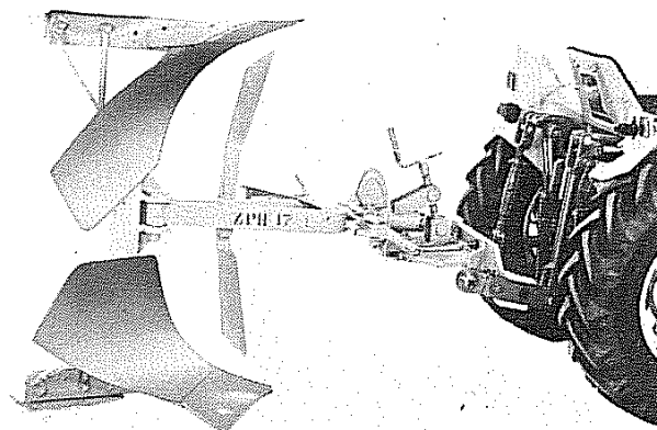
Fig. 90 - Aratro voltaorecchio a 180° mod. "ZPH17"
