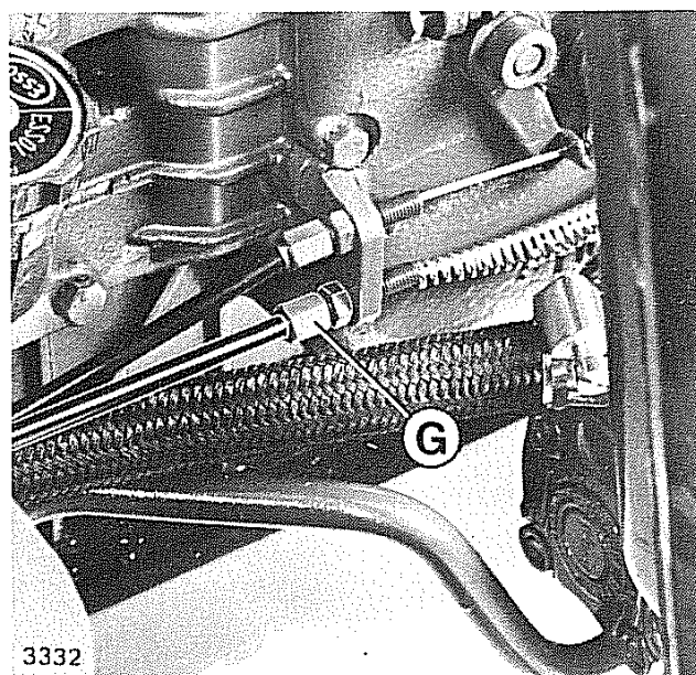
Fig. 39 - Registrazione arresto motore mod. 526T
