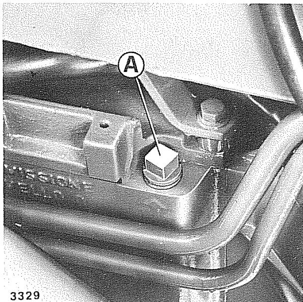
Fig. 23 - Immissione e livello olio nel carter cambio
