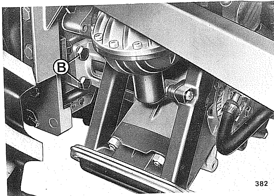
Fig. 103 - Attacco pompa
