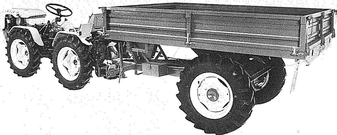
Fig. 49 - Rimorchio a ruote motrici mod. "C52"
