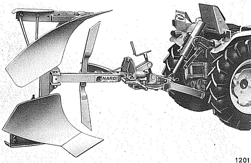
Fig. 61 - Aratro voltaorecchio a 180° mod. "ZPH17"
