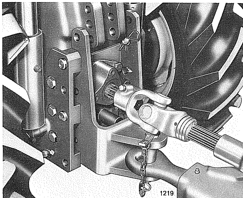
Fig. 81 - Attacco rimorchi mod. "C58" e "C59"
