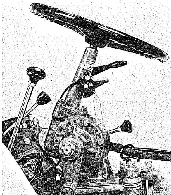
Fig. 16 - Sterzo meccanico
