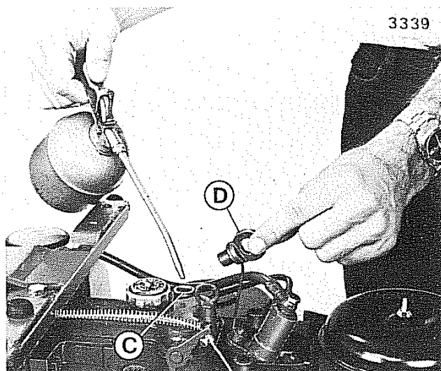
Fig. 18 - Supplemento a olio
