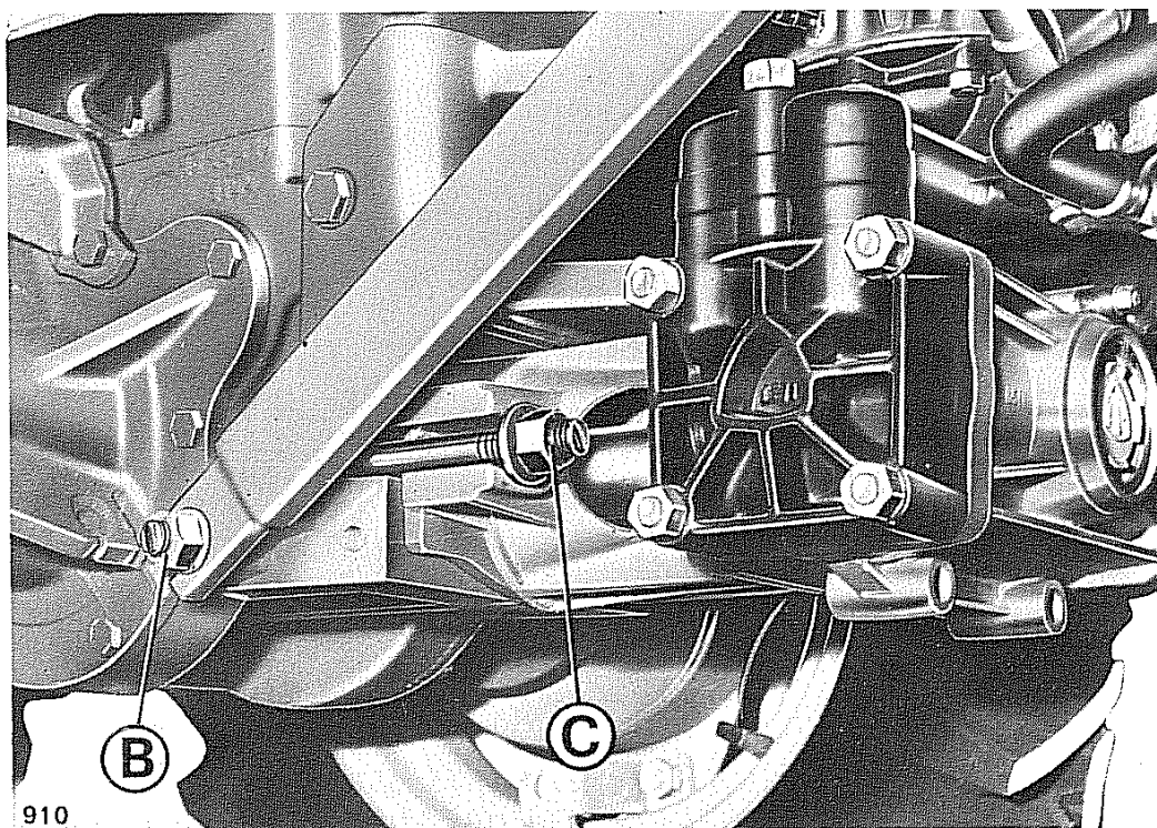
Fig. 67 - Attacco pompa
