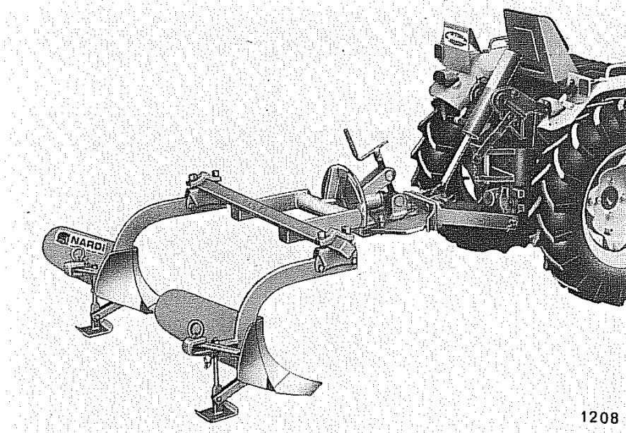
Fig. 62 - Assolcatore-Rincalzatore mod. "2AS13"
