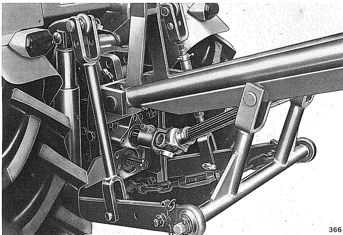
Fig. 109 - Attacco trivella
