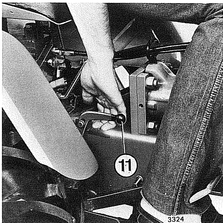
Fig. 12 - Innesto presa di forza sincronizzata
