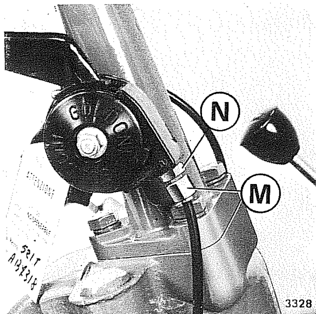
Fig. 42 - Registrazione manettino acceleratore
