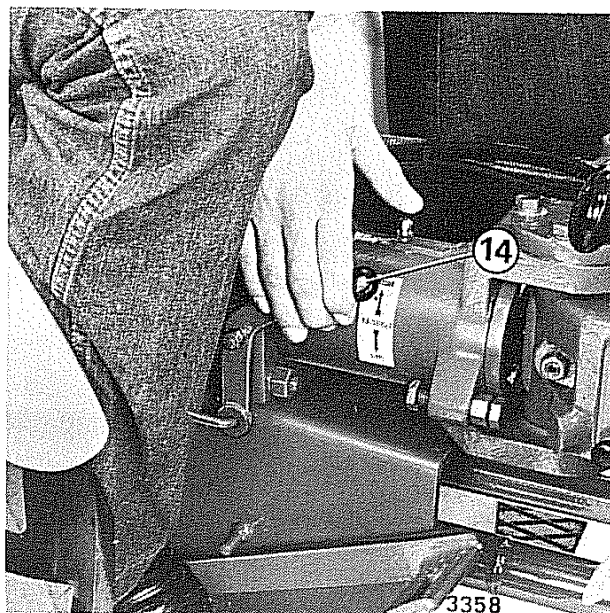
Fig. 10 - Bloccaggio differenziale posteriore
