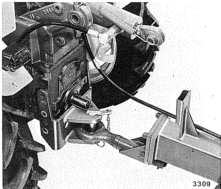
Fig. 48 - Attacco rimorchio mod. "C44/1"
