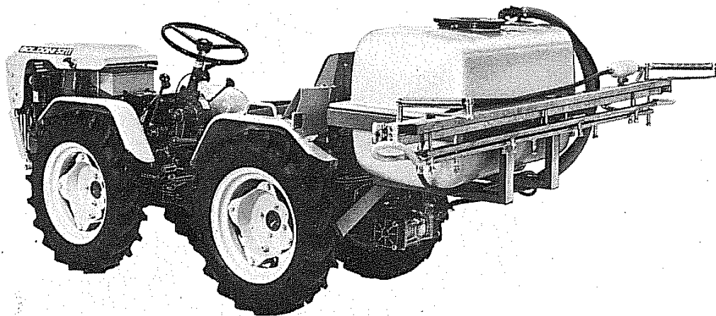
Fig. 65 - Gruppo diserbante
