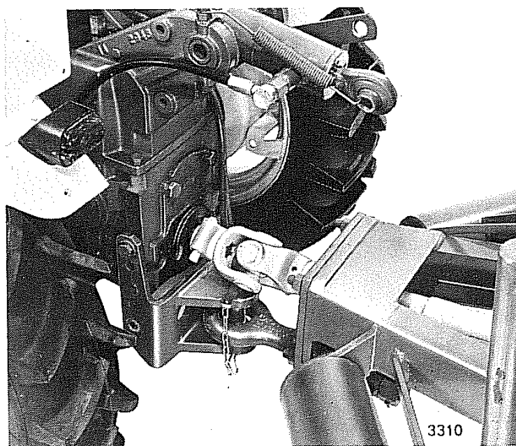
Fig. 50 - Attacco rimorchio mod. "C52"
