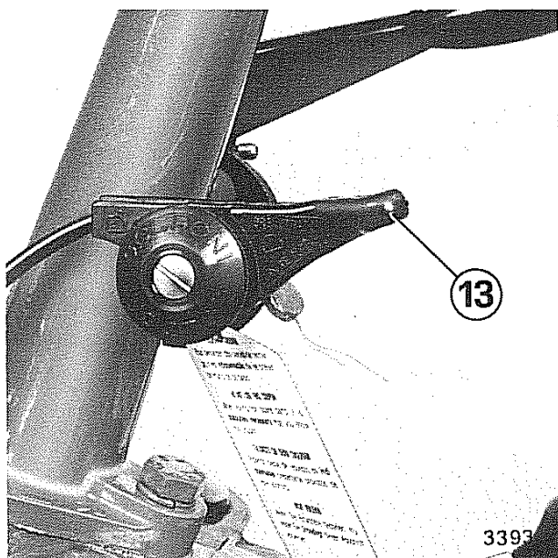
Fig. 2 - Arresto motore per mod. 526T e 530T.
