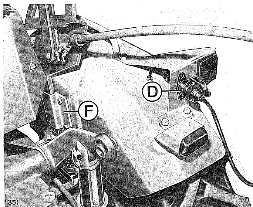
Fig. 82 - Attacco spina e leva freno
