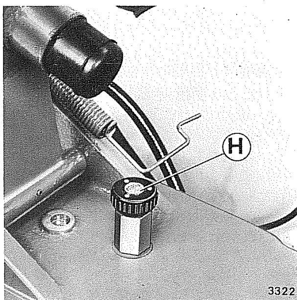
Fig. 29 - Sfiato olio nel sollevatore a 2 punti
