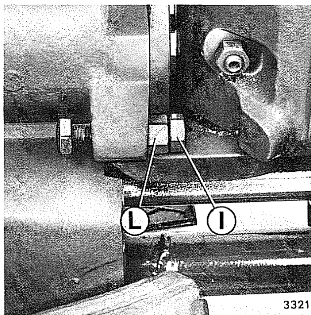
Fig. 41 - Registrazione raggio di sterzata
