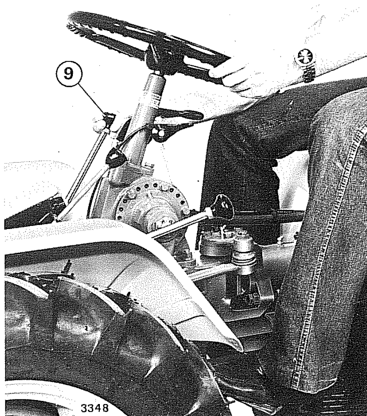
Fig. 7 - Innesto delle velocità
