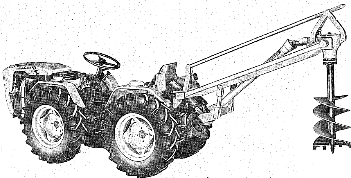
Fig. 72 - Trivella
