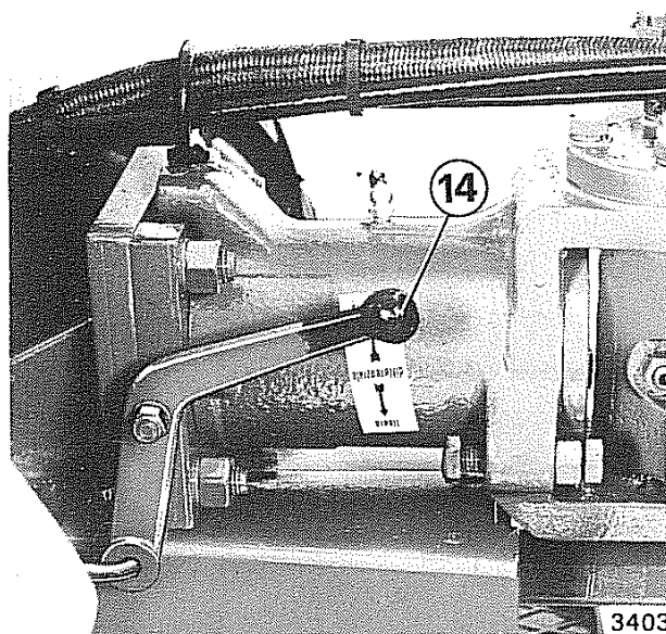
Fig. 3 - Bloccaggio differenziale posteriore.
