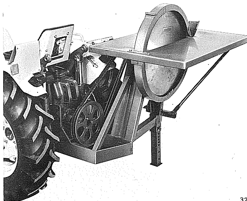
Fig. 105 - Sega circolare
