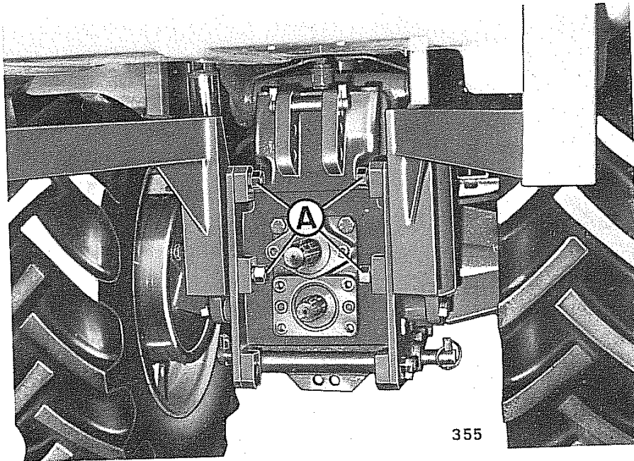
Fig. 102 - Attacco fusto
