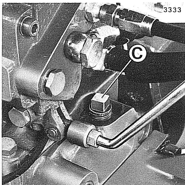
Fig. 25 - Immissione e livello olio nel differenziale posteriore
