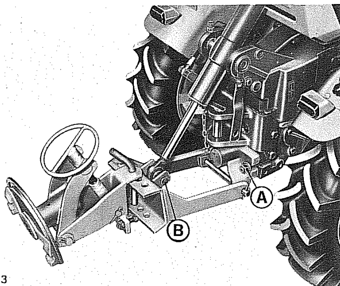
Fig. 53 - Porta aratri mod. "P13"
