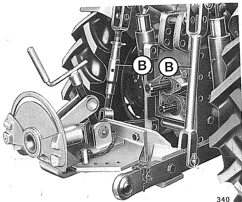
Fig. 84 - Porta aratri mod. "PH17"
