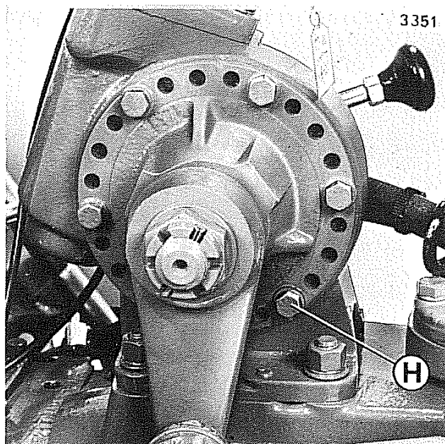
Fig. 40 - Registrazione sterzo
