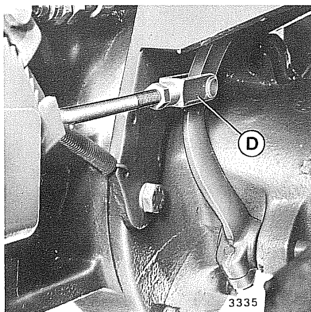
Fig. 37 - Registrazione freni di soccorso e stazionamento
