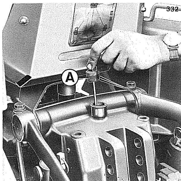
Fig. 30 - Immissione e livello olio nel sollevatore a 3 punti
