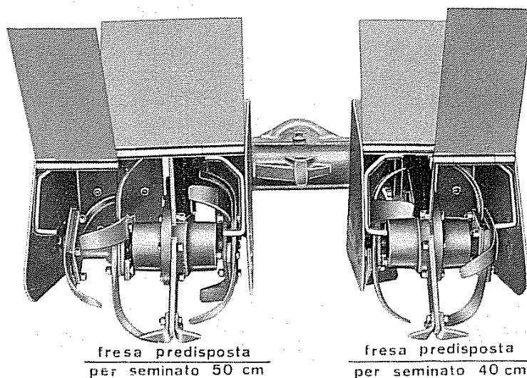
Fig. 2 - Regolazione larghezza fresa
