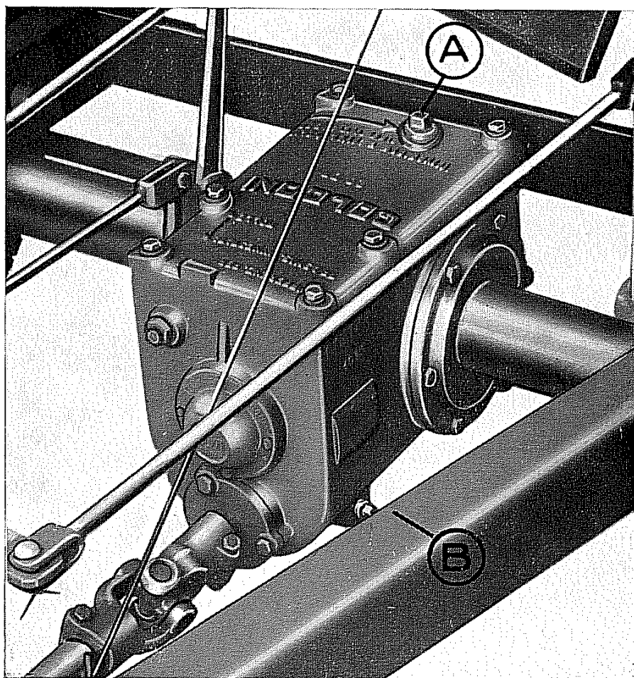
Fig. 1 - Sostituzione olio
